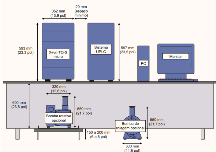
Figura 2 – Vista frontal, mostrando os requisitos de espaço
