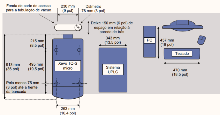
Figura 1 – Vista plana, mostrando os requisitos de espaço
